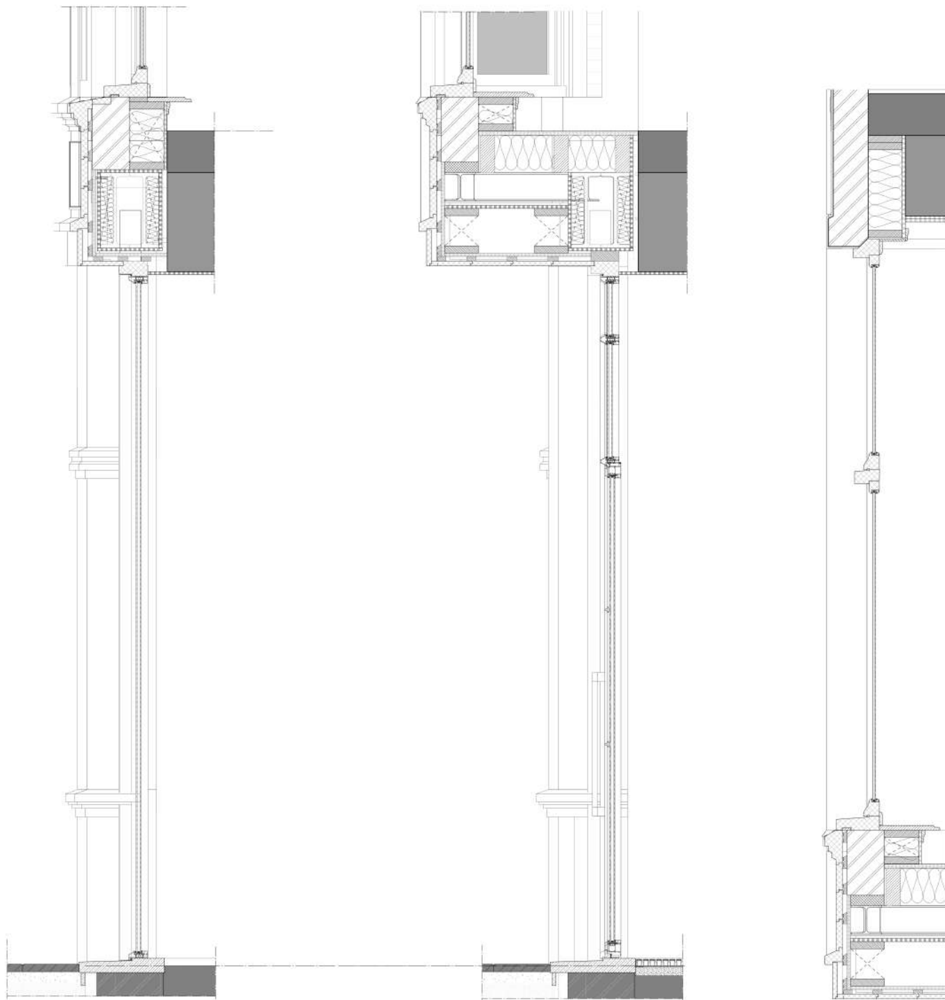
Herestraat 72 - Detaillering
