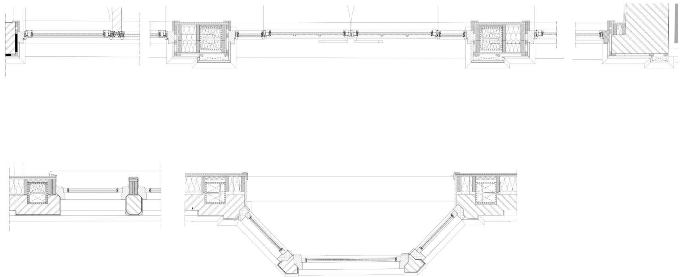
Herestraat 72 - Detaillering
