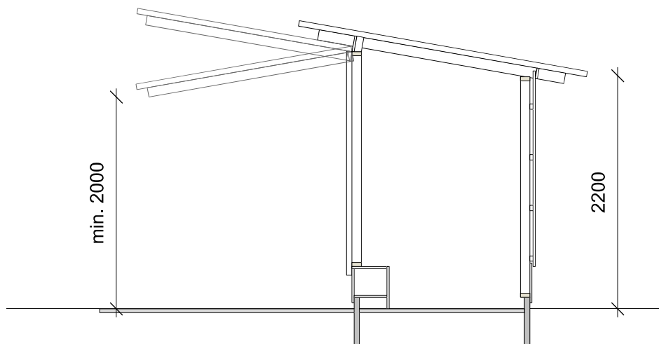
Doorsnede
