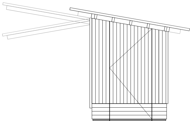
Zijgevel (rechts)
