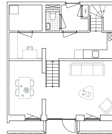
Tussen maisonnettes
